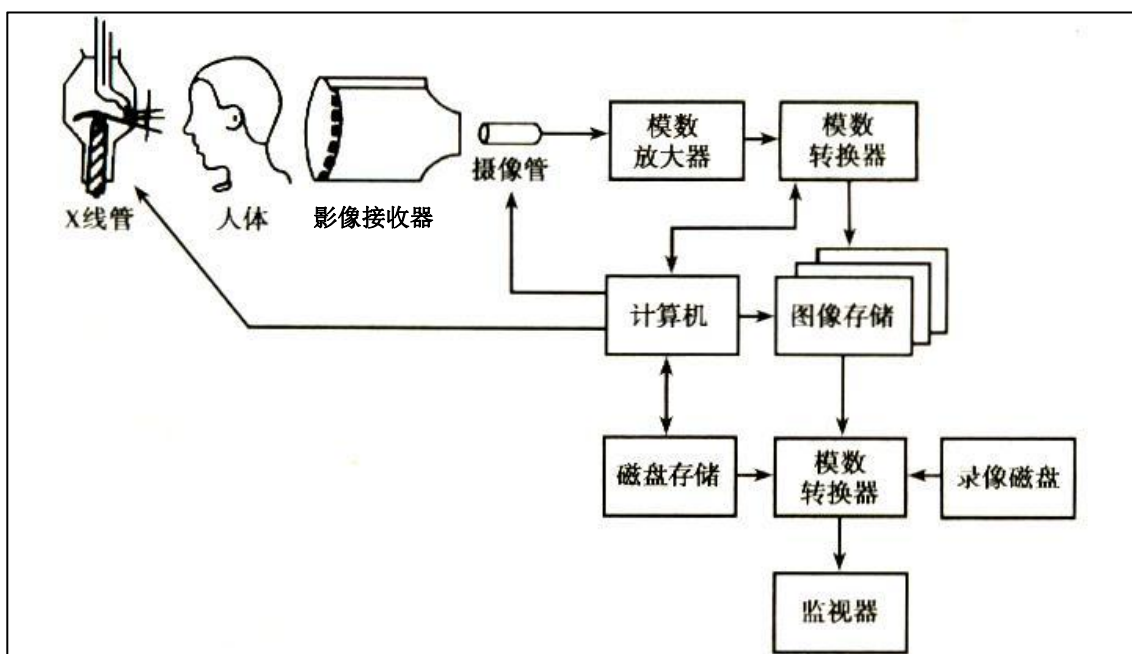
图 9-3 DSA 系统结构图
