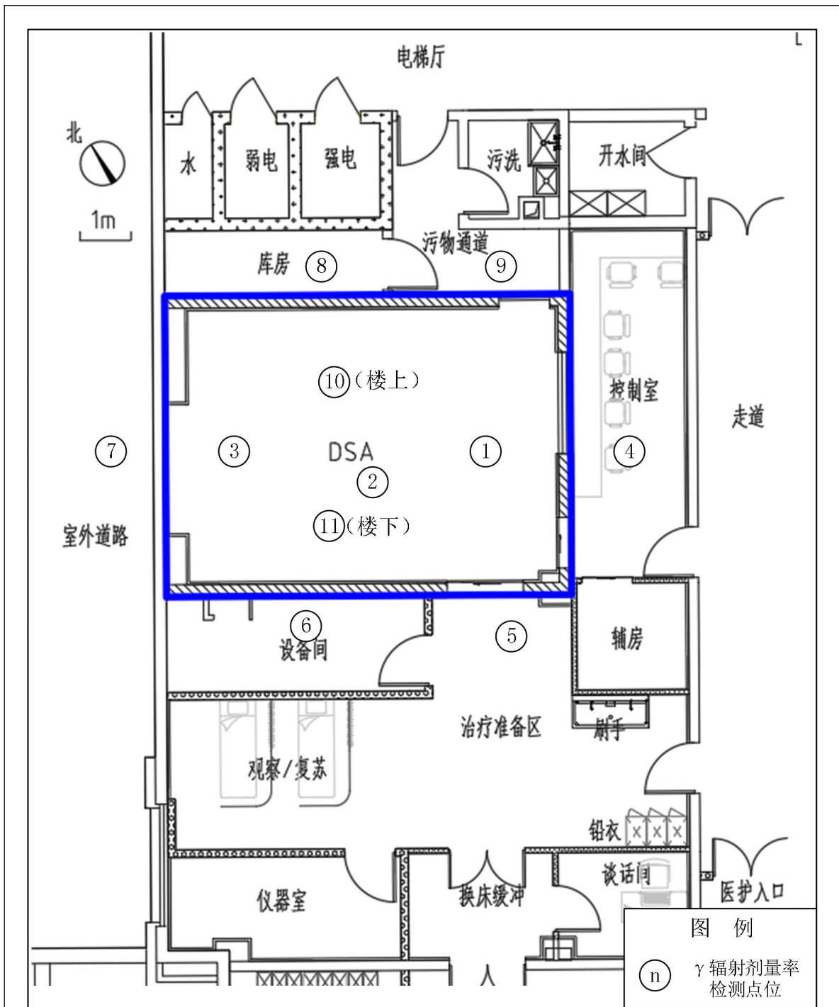
图 8-7 常州市第二人民医院搬迁 1 台 DSA 项目现场检测点位平面示意图 (1)
