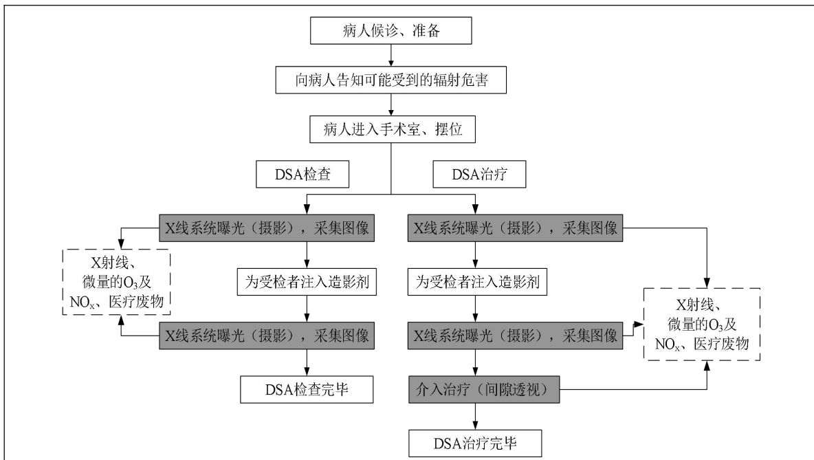
图 9-4 本项目 DSA 工作流程及产污环节示意图
