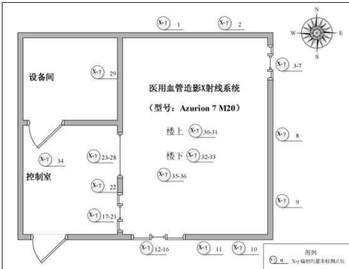
图 7-1 DSA 室周围 X-γ辐射剂量率检测点位示意图
