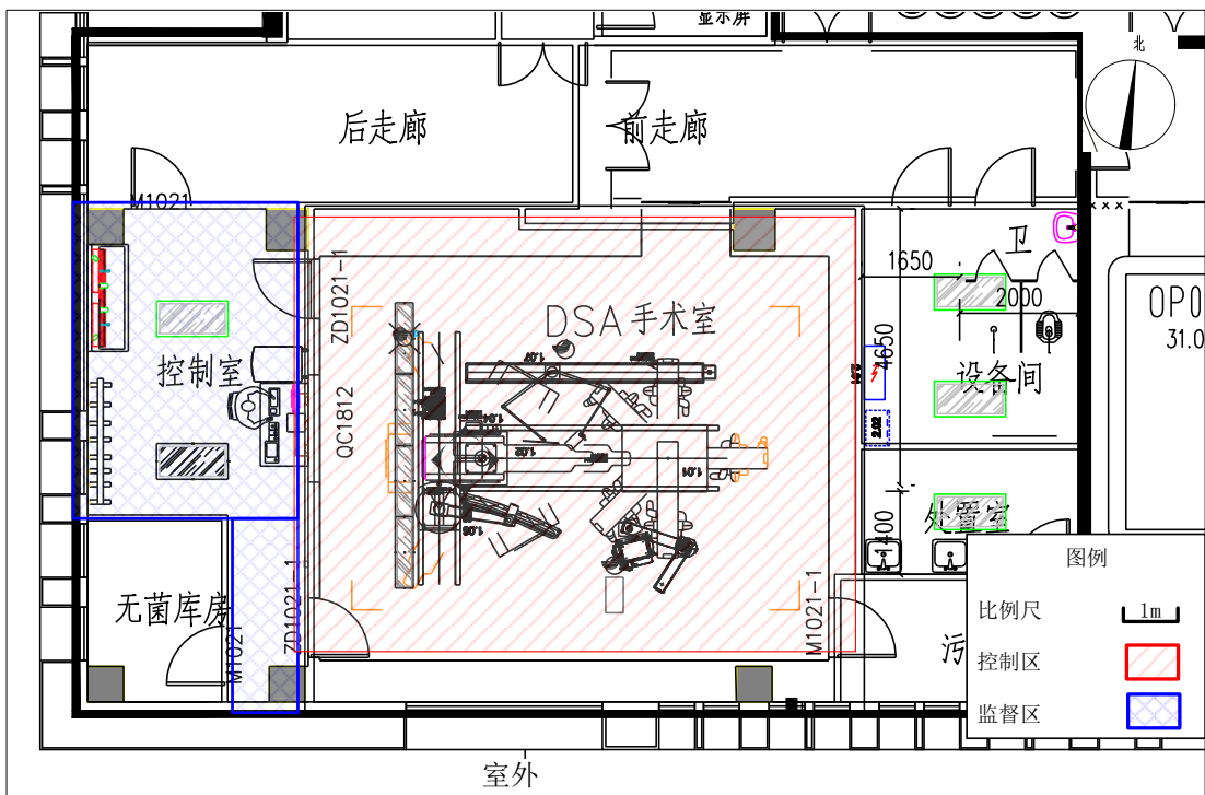
图3-2 本项目DSA机房平面布置及分区示意图
