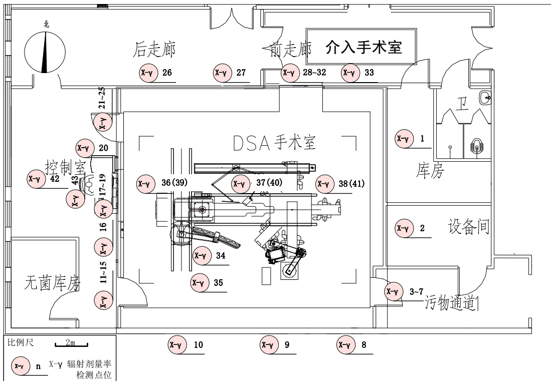
图7-1 本项目DSA机房周围X-γ辐射剂量率监测布点图
