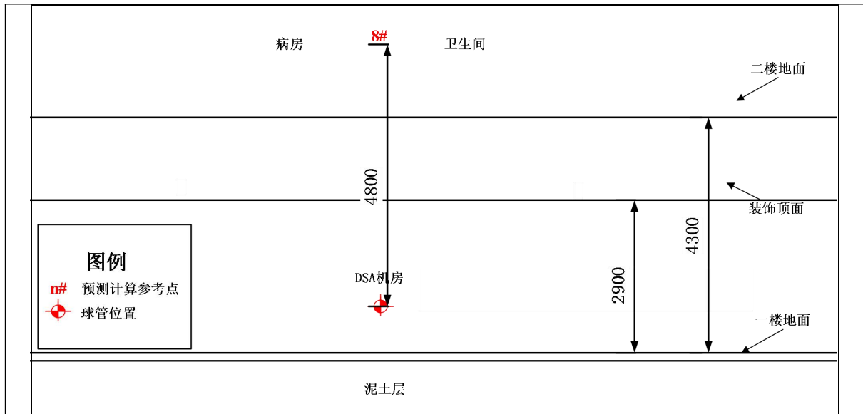
图 11-2 DSA 机房预测点布设剖面示意图
