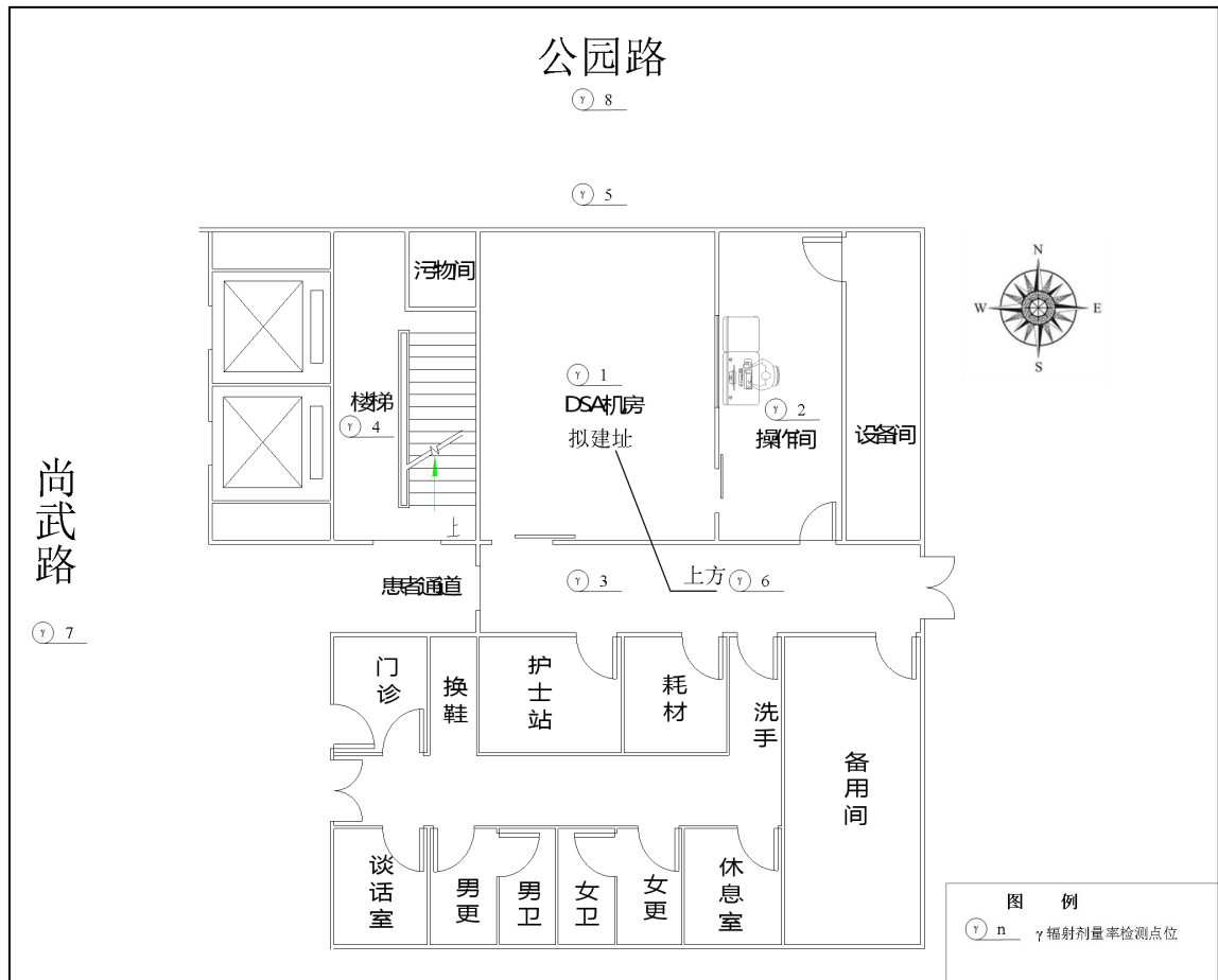
图 8-7 沛县敬安镇中心卫生院新增 1 台 DSA 项目拟建址周围环境 \gamma 辐射监测点位示意图
