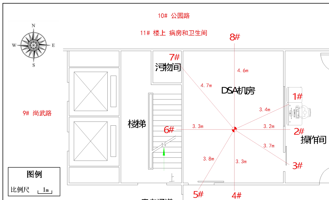
图 11-1 DSA 机房周围预测点布设示意图
