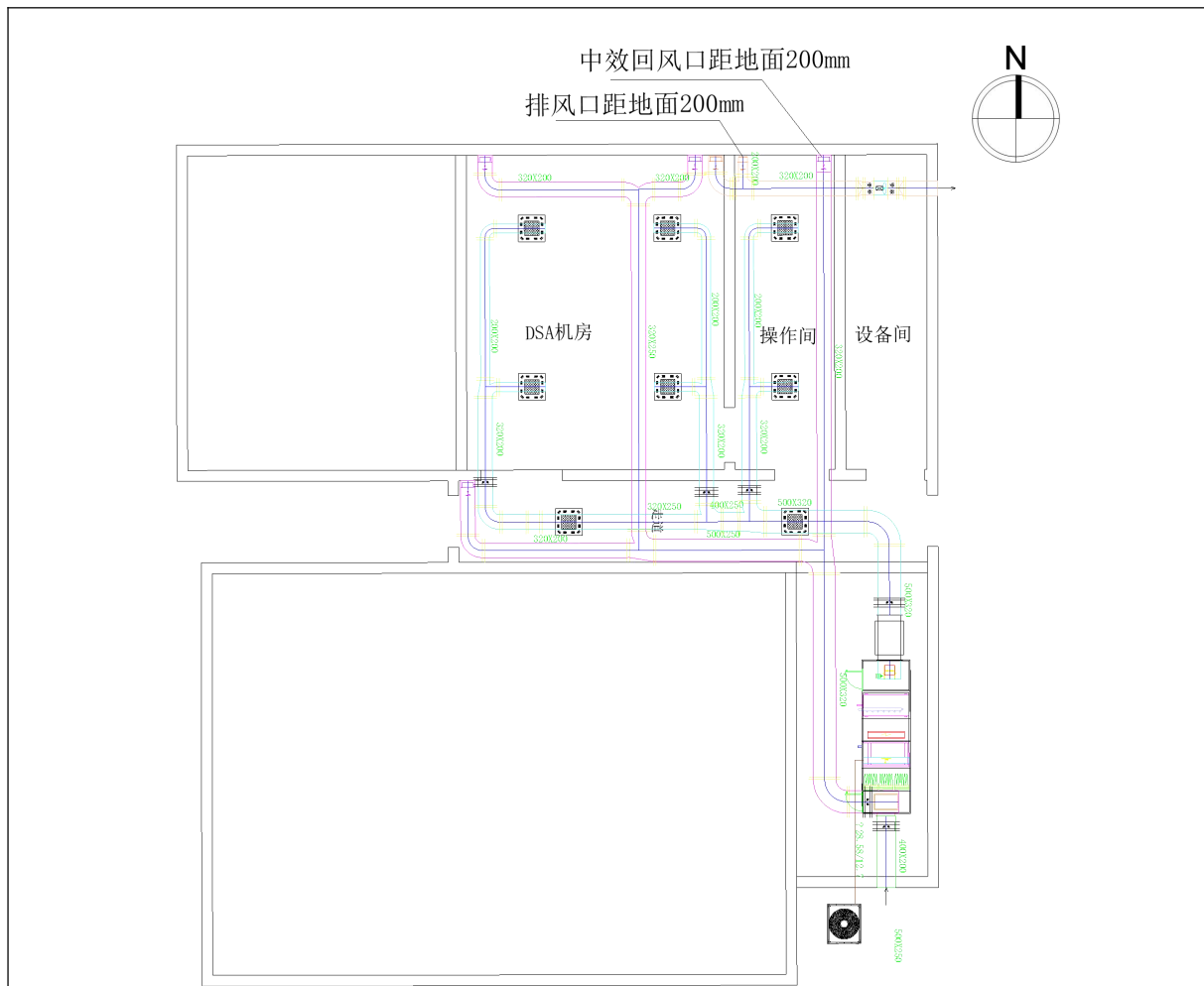
图 10-3 本项目 DSA 机房通风设计示意图
