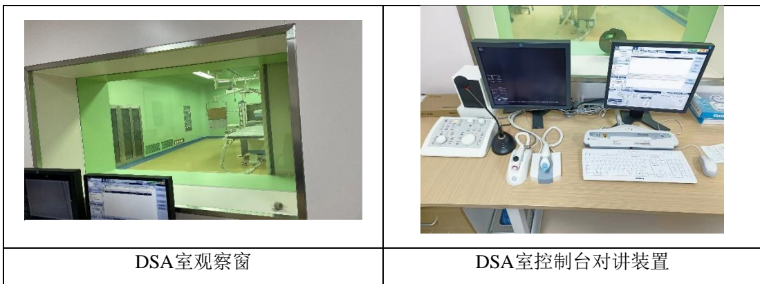
图3-3 本项目DSA机房观察窗及对讲装置
