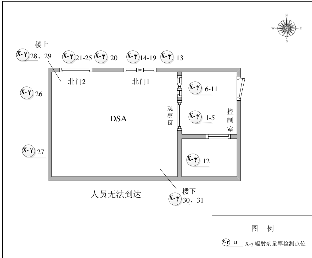
图7-1 病房楼二楼介入科DSA室周围监测布点图
